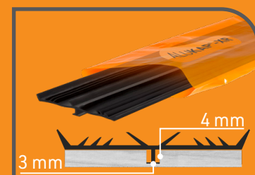
Joint de chevron à gorge 55 mm
